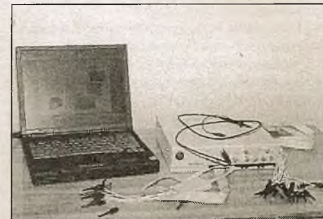
Распрацоўка факультэта: прыстаўка да персанальнага камп'ютэра прыдае яму функцыі вымяральных прыладаў (лічбавая асцыляграф, генератар сігналаў адвольнай формы, шматканальнага лагічнага аналізатара)
